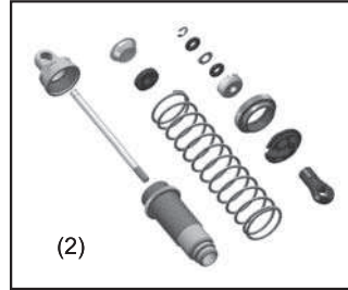
PD7729 REAR ALUM*SHOCK SET 後鋁合金避震器組
