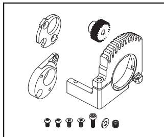
PD9269 MOTOR MOUNT 馬達固定座
