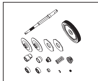
PD9223 SLIPPER CLUTCH SET 扭力限制組
