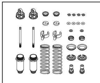
PD9266 FRONT SHOCK SET 前避震器組
