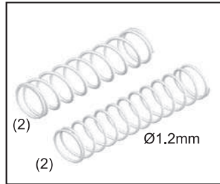
PD7721-W SHOCK SPRING(W) 避震器彈簧組(白)
